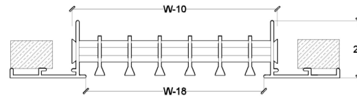
LINEAR BAR GRILLE RETURN
