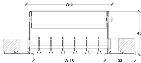
LINEAR BAR BLADE GRILLE (LBBG)
